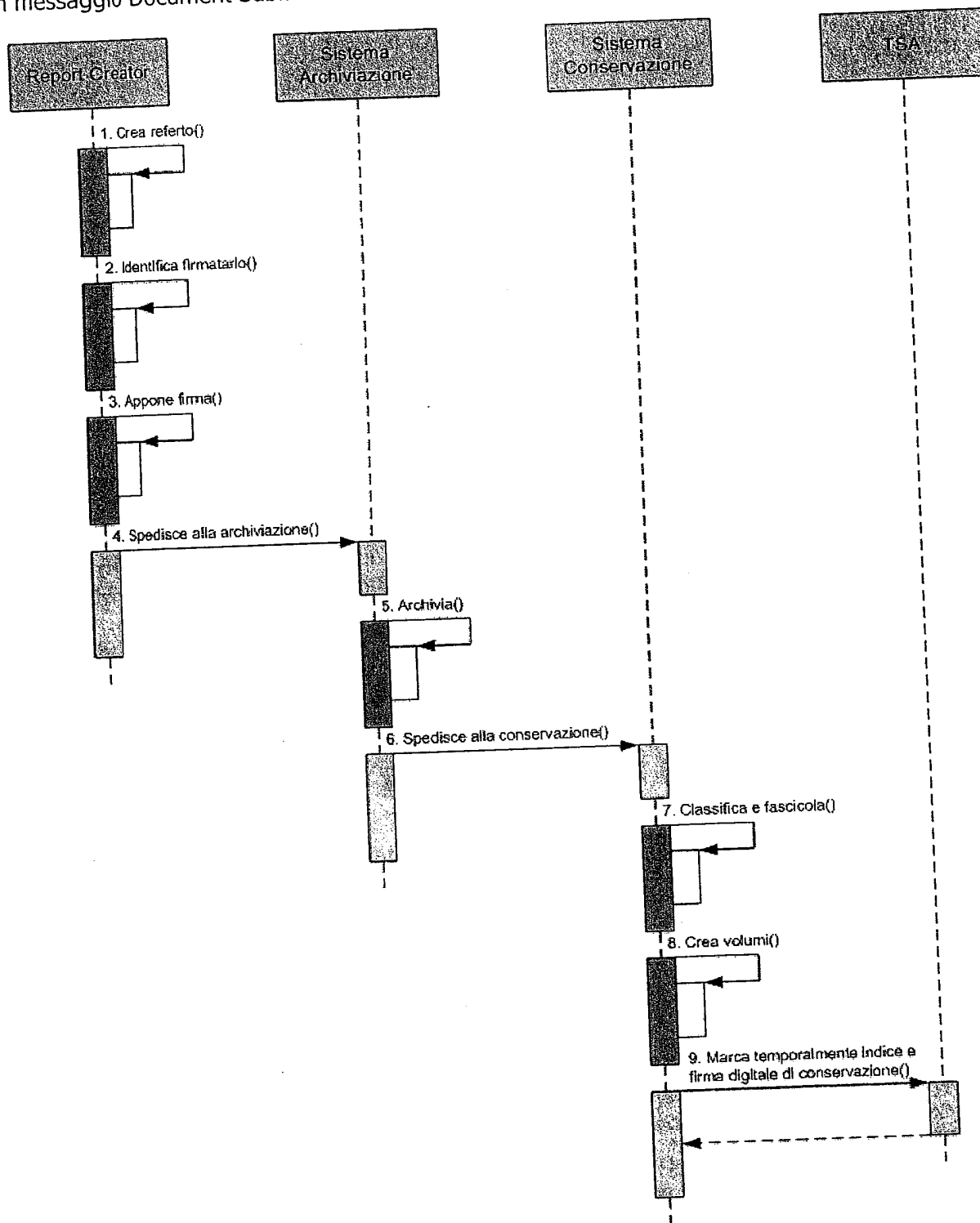
Figura 9.1: diagramma di sequenza del processo di dematerializzazione
